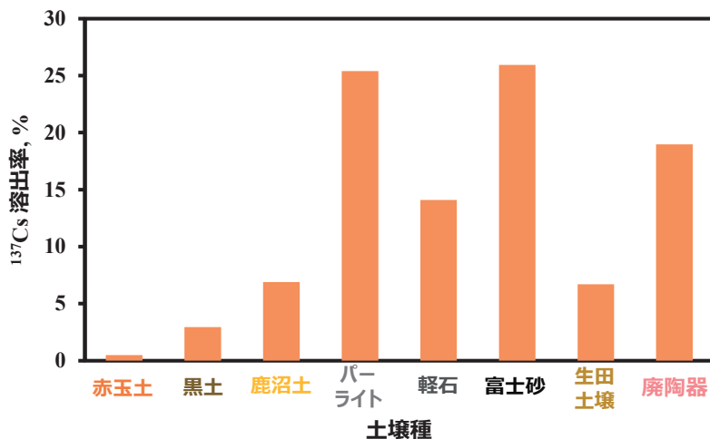
図3 都市ごみ焼却飛灰・土壤混合GS体からの ^{137}\text{Cs} 溶出率。
