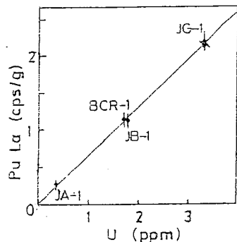
図2. Uの検量線(横軸は文献値)
