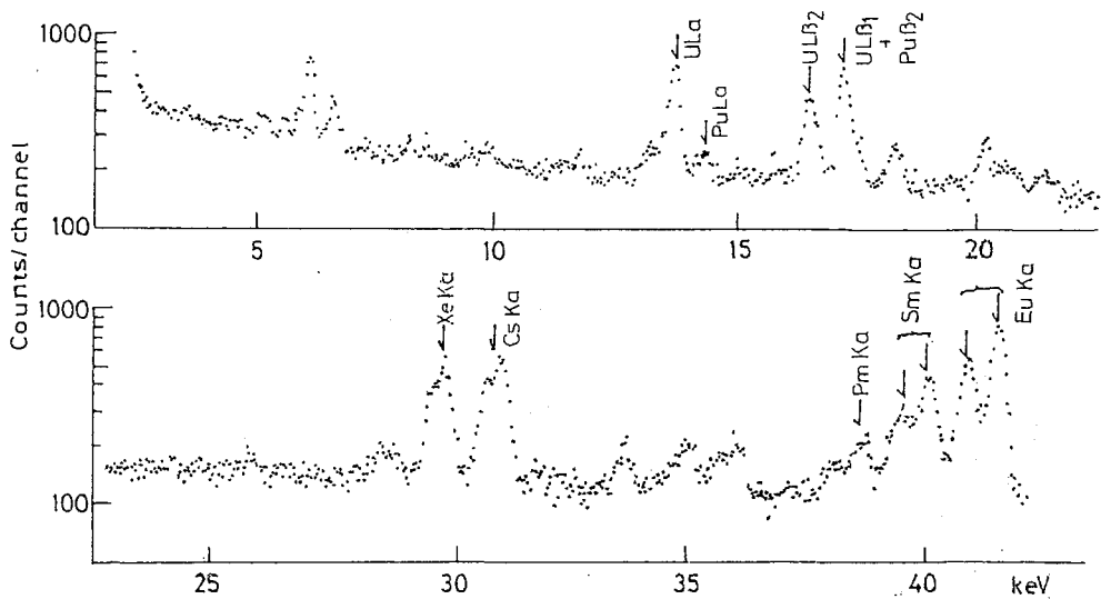
図1. JB-1のX線スペクトル(24h照射, 11d冷却, 40000s測定)
