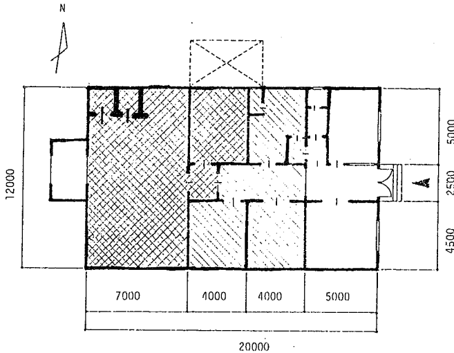
図1 トリチウム取扱実験棟のゾーニング
