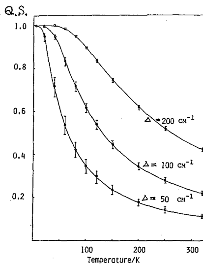
図3. T_d Symmetryで d_{x^2-y^2} , d_{z^2} 軌道のエネルギー差 \Delta としに各 \Delta での四極分岐の温度変化を示しに。縦棒は \Delta に \pm 5 \text{ cm}^{-1} の変化があったときの变化値を示す。
