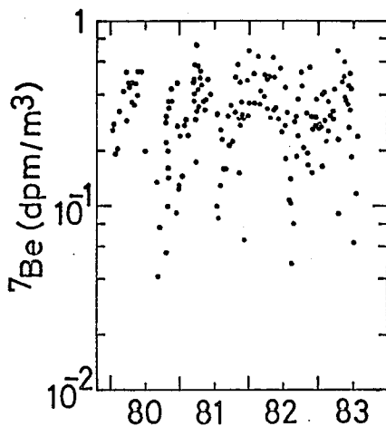
図2 大気中における ^7\text{Be} 濃度の時間変化
